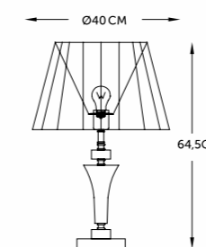
1044 Abajur Belinda Base Cristal Cúpula Café 1*E27 60W Ø40*64,5cm
