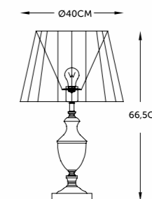
1046 Abajur Birgit Base Cristal Cúpula Café 1*E27 60W Ø40*66,5cm
